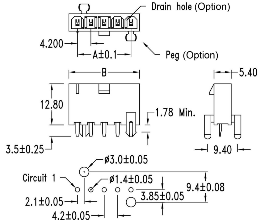
P.C.B. hole dimensions
