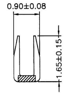
SEC A-A
