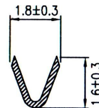
A-A SECTION
