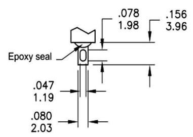
SOLDER LUG
