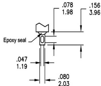
SOLDER LUG
