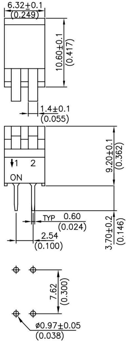
P.C.B. LAYOUT
