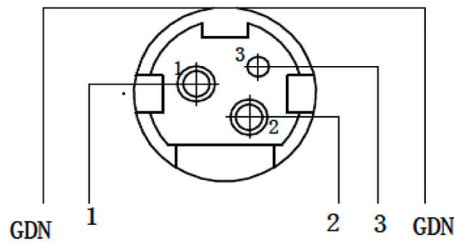
电路图
