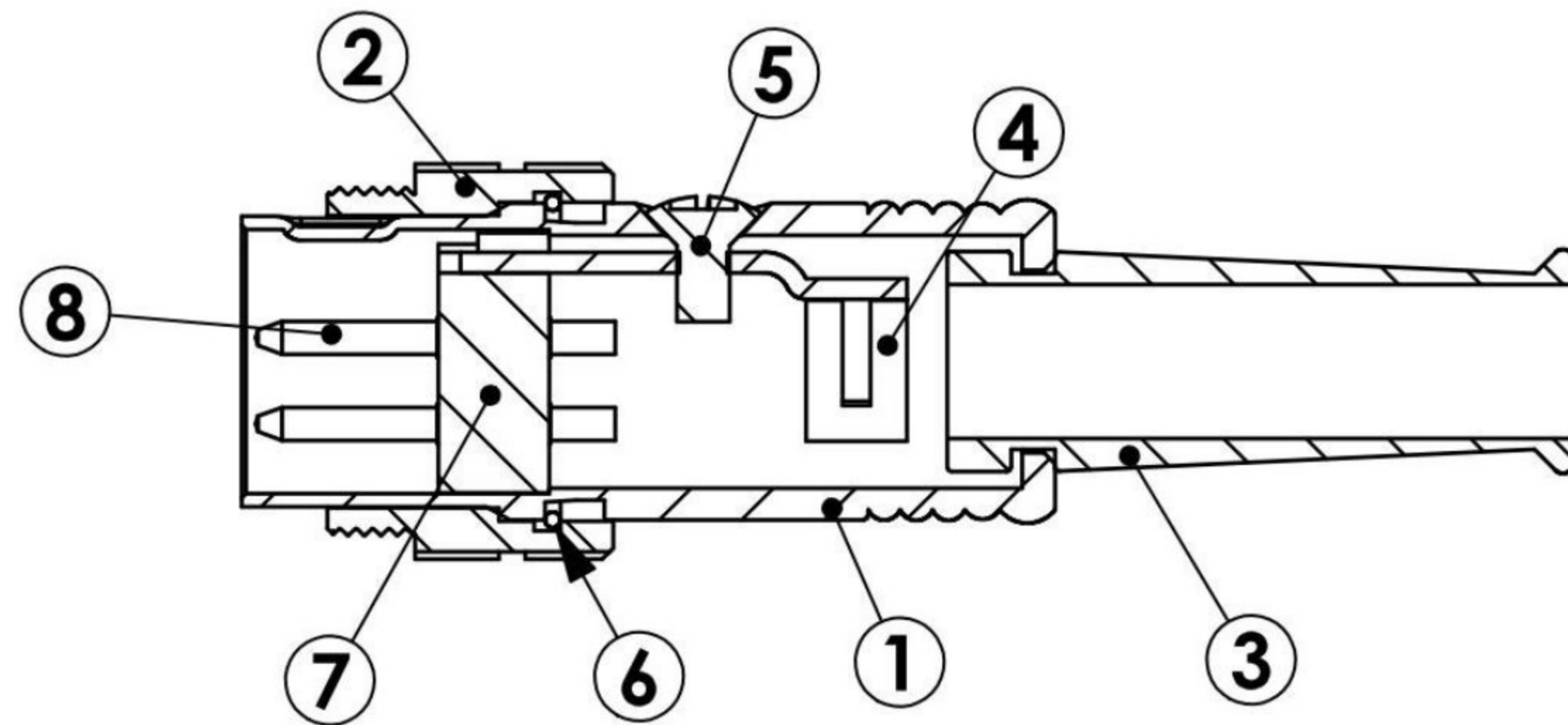
A-A SECTION
