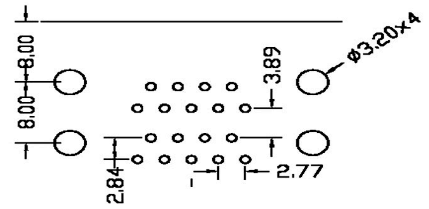
P. C. B LATOUT
