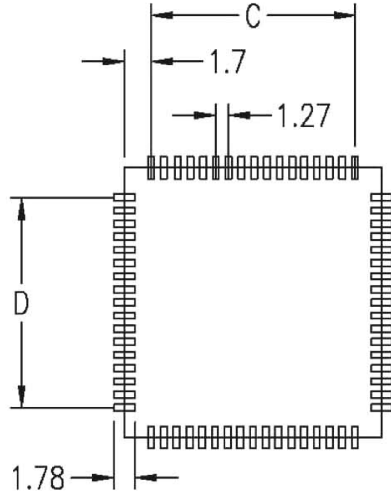
P.C.B LAYOUT
