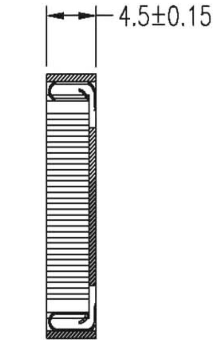
SECTION A-A
