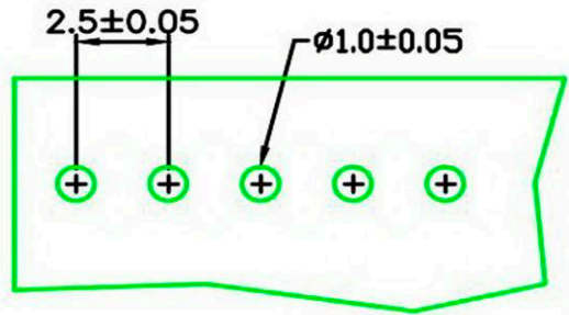
P.C.BOARD LAYOUT
