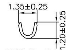
SEC:B-B
