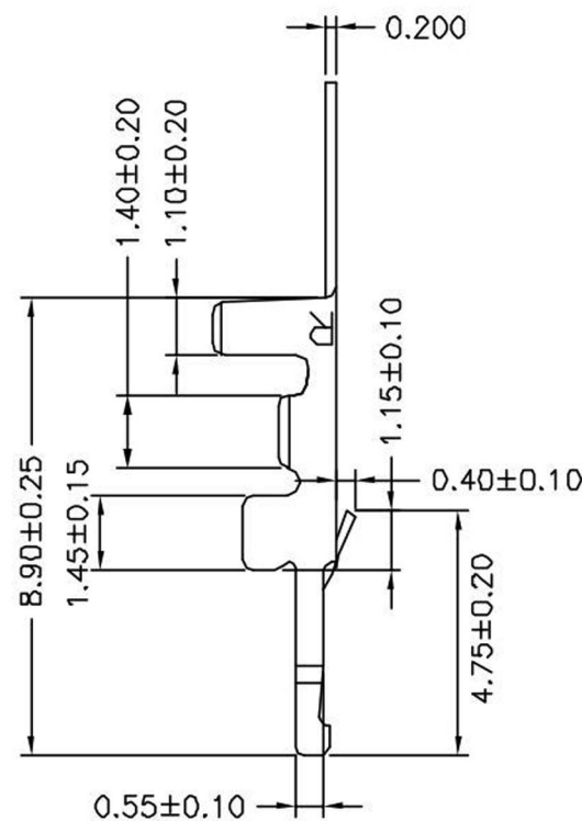
SEC:A-A
